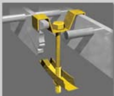
ÍTEM 28: Sujeción estándar con lomo, perno, tuercas y arandela para fijar de forma segura le parte superior e inferior.
